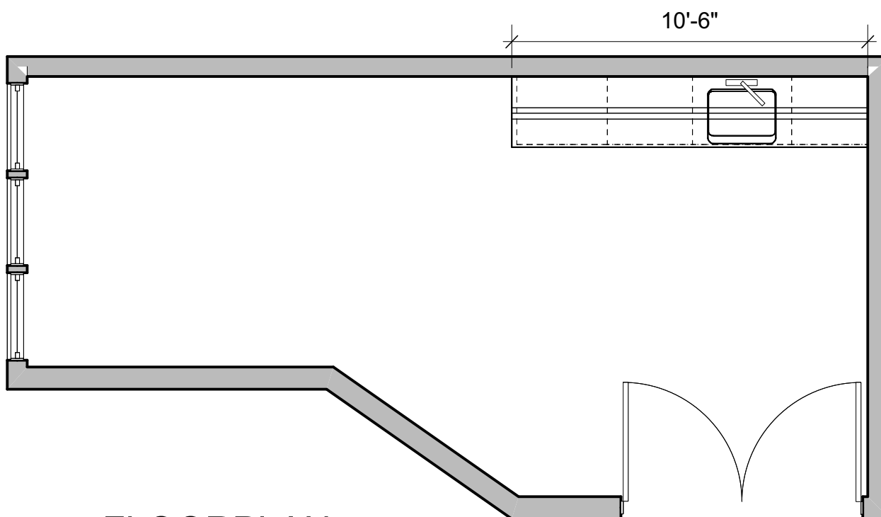
1 FLOORPLAN Scale: 1/4" = 1'-0"
